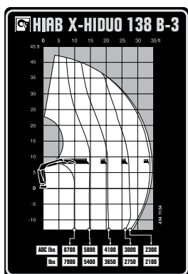
HIAB X-HIDUO 138B-3
