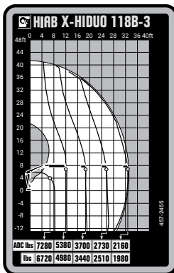
HIAB X-HIDUO 118B-3
