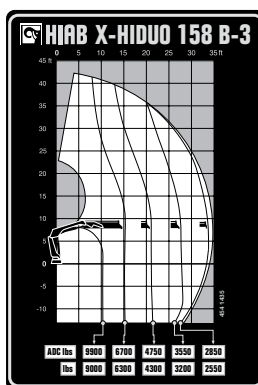
HIAB X-HIDUO 158B-3
