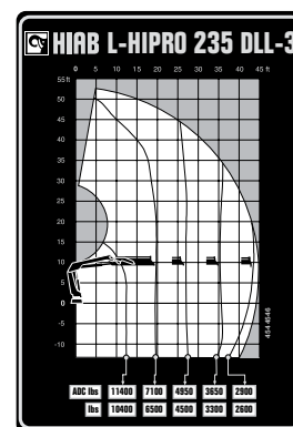
HIAB L-HIPRO 235 DLL-3
