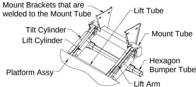
RZ-10 RZ-20
